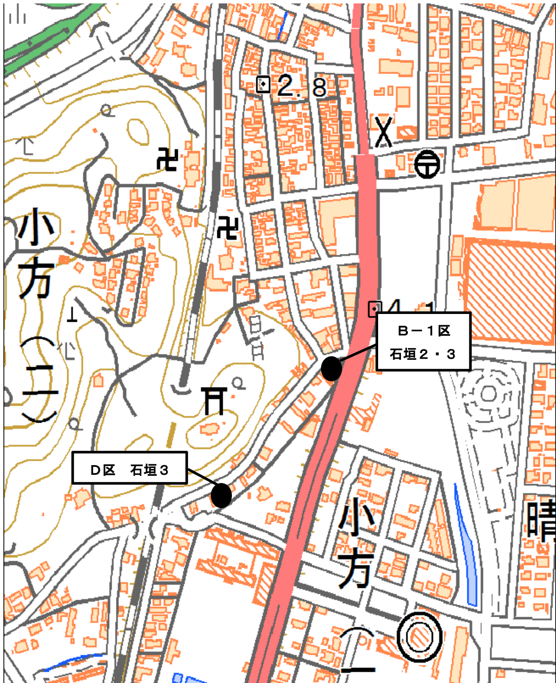
亀居城関連遺跡 石垣測量石垣位置図
