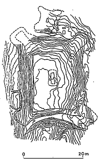
小羽山30号墓 (福井市)
