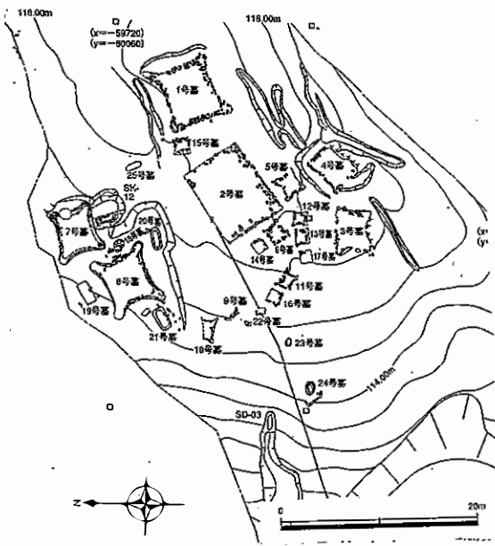
洞ノ原墳墓群 (米子市・大山町)
